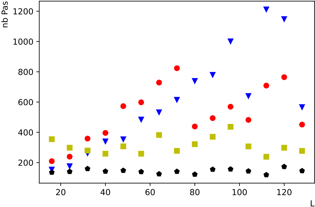
Estimation du nombre de pas Monte Carlo à effectuer pour atteindre la stabilisation Condition Initiale aléatoire
